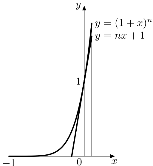
Рис. 1. График функции y = (1+x)^n и касательная к нему y = nx + 1 .
